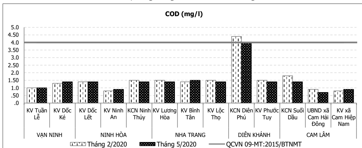
Biểu đồ 2.12. Diễn biến COD trong nước dưới đất 6 tháng đầu năm 2020
