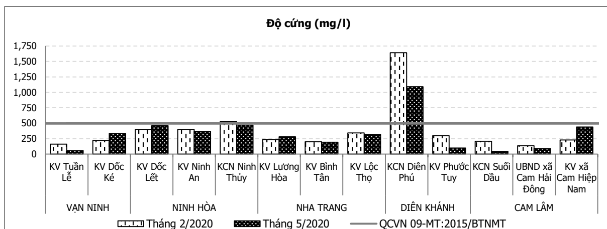
Biểu đồ 2.11. Diễn biến độ cứng trong nước dưới đất 6 tháng đầu năm 2020
