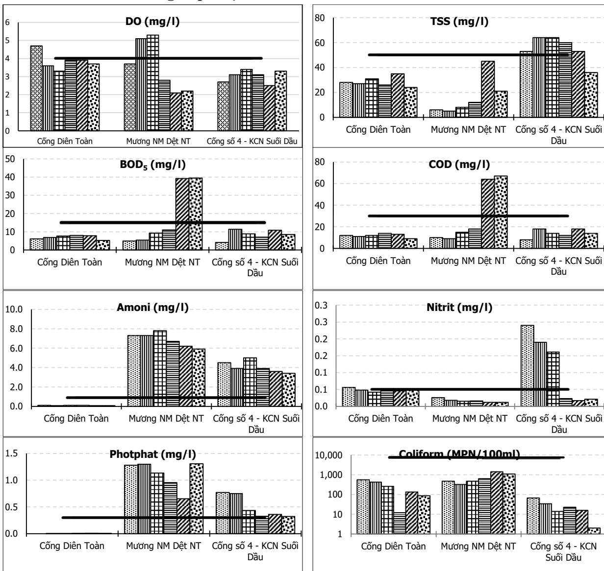
Biểu đồ 2.9. Diễn biến chất lượng nước tại các kênh mương 6 tháng đầu năm 2020
