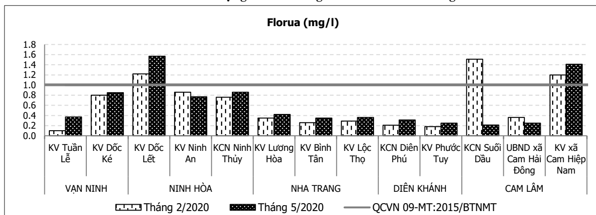
Biểu đồ 2.14. Diễn biến hàm lượng florua trong nước dưới đất 6 tháng đầu năm 2020
