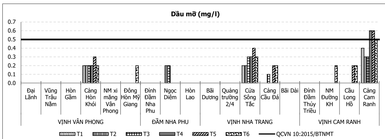
Biểu đồ 2.21. Diễn biến giá trị Dầu mỡ trong nước biển ven bờ 6 tháng đầu năm 2020
