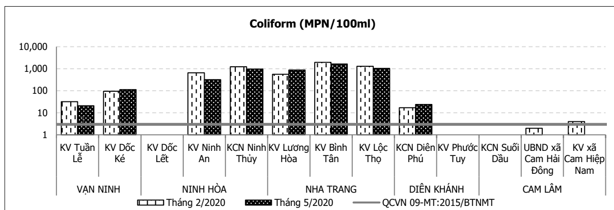
Biểu đồ 2.17. Diễn biến mật độ coliform trong nước dưới đất 6 tháng đầu năm 2020
