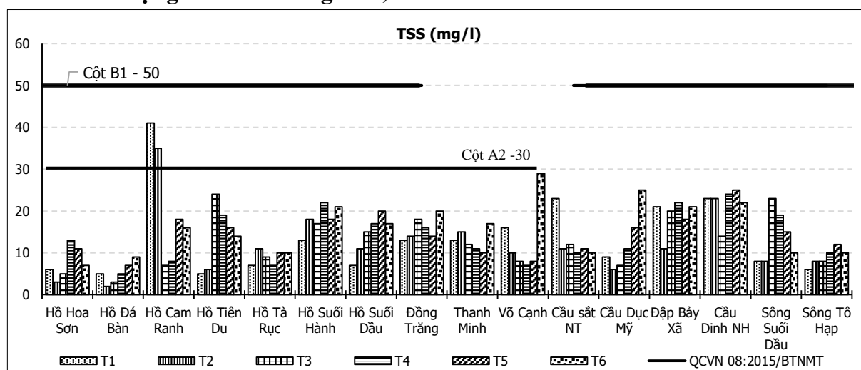
Biểu đồ 2.3. Diễn biến hàm lượng TSS tại các hồ chứa và sông suối 6 tháng đầu năm 2020
