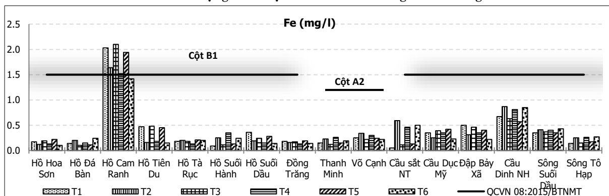
Biểu đồ 2.7. Diễn biến hàm lượng Fe tại các hồ chứa và sông suối 6 tháng đầu năm 2020
