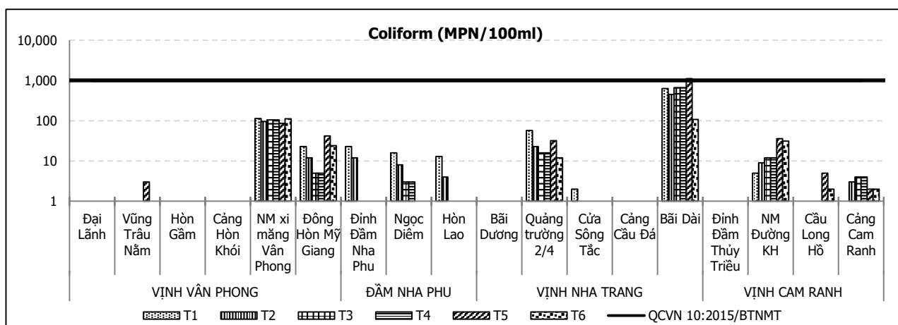
Biểu đồ 2.22. Diễn biến giá trị Coliform trong nước biển ven bờ 6 tháng đầu năm 2020
