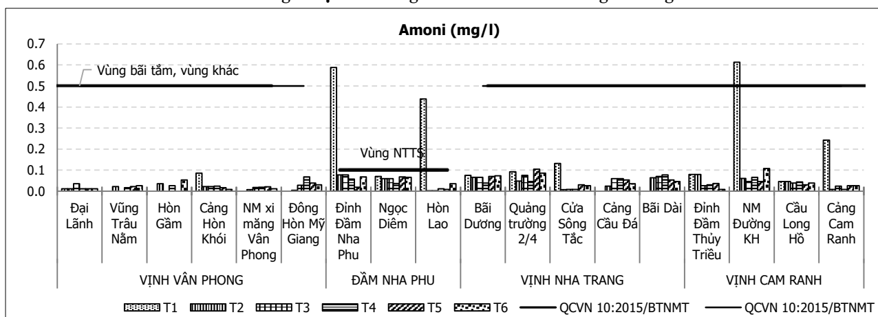
Biểu đồ 2.20. Diễn biến giá trị Amoni trong nước biển ven bờ vùng 6 tháng đầu năm 2020
