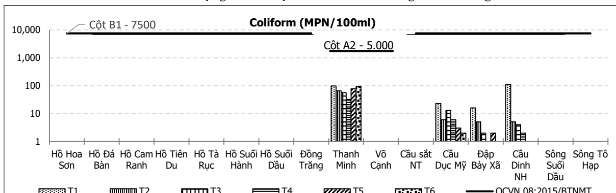
Biểu đồ 2.9. Diễn biến hàm lượng Coliform tại các hồ chứa và sông suối 6 tháng đầu năm 2020
