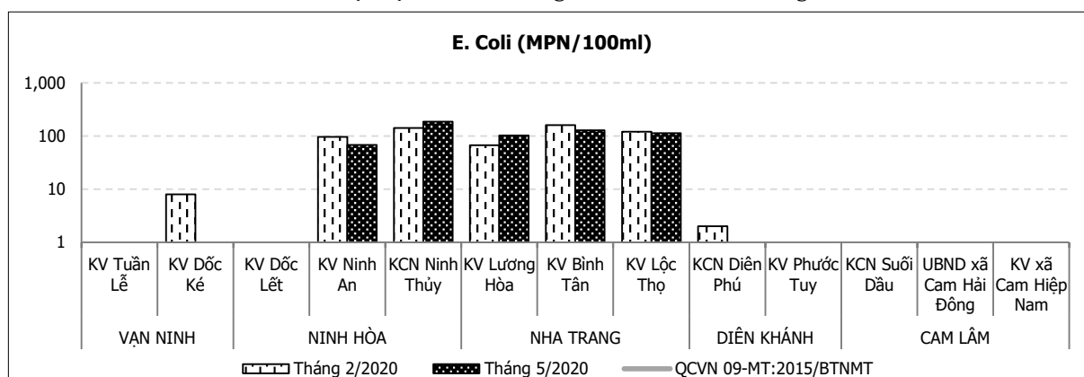
Biểu đồ 2.18. Diễn biến mật độ coliform trong nước dưới đất 6 tháng đầu năm 2020
