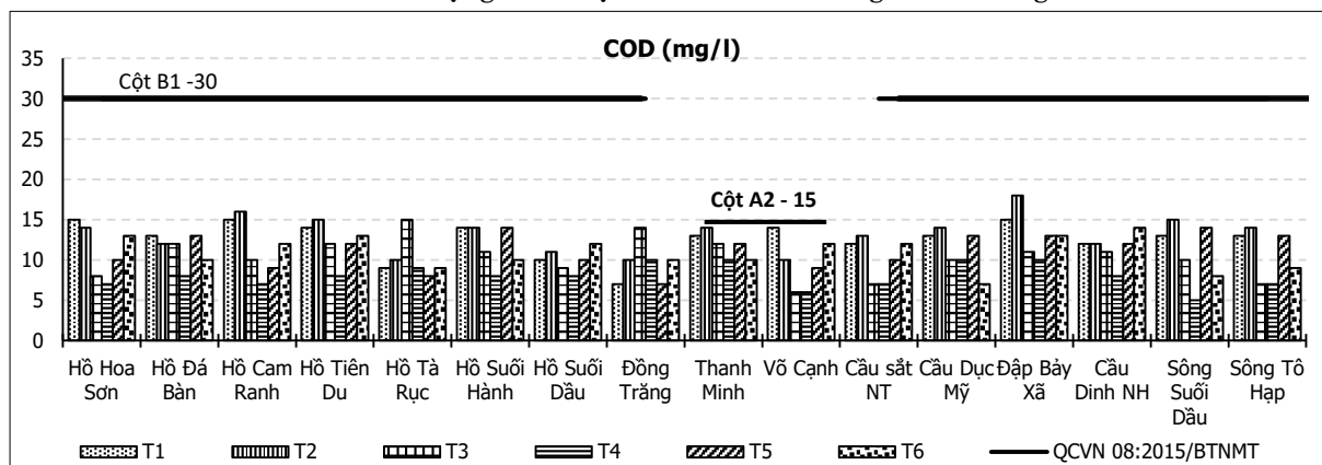
Biểu đồ 2.5. Diễn biến hàm lượng COD tại các hồ chứa và sông suối 6 tháng đầu năm 2020
