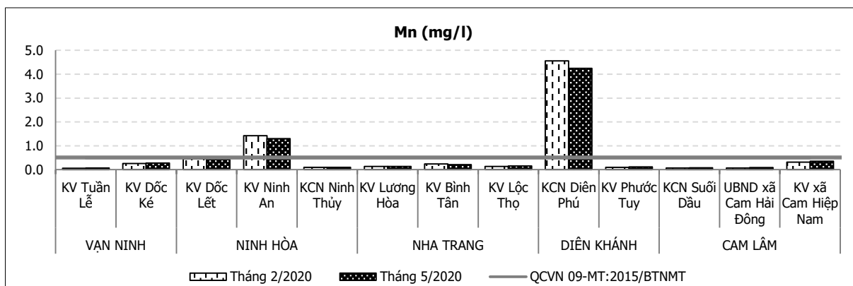
Biểu đồ 2.16. Diễn biến hàm lượng Mn trong nước dưới đất 6 tháng đầu năm 2020
