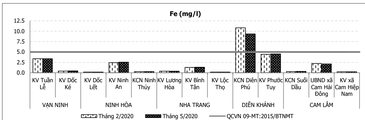
Biểu đồ 2.15. Diễn biến hàm lượng Fe trong nước dưới đất 6 tháng đầu năm 2020
