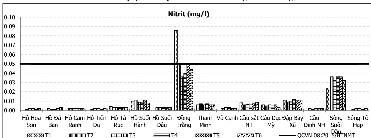
Biểu đồ 2.6. Diễn biến hàm lượng Nitrit tại các hồ chứa và sông suối 6 tháng đầu năm 2020
