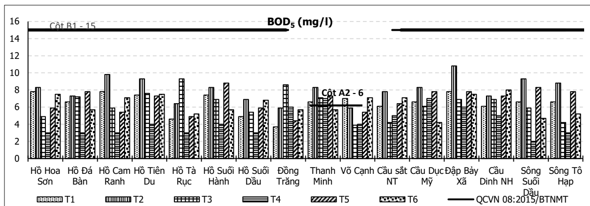
Biểu đồ 2.4. Diễn biến hàm lượng BOD 5 tại các hồ chứa và sông suối 6 tháng đầu năm 2020
