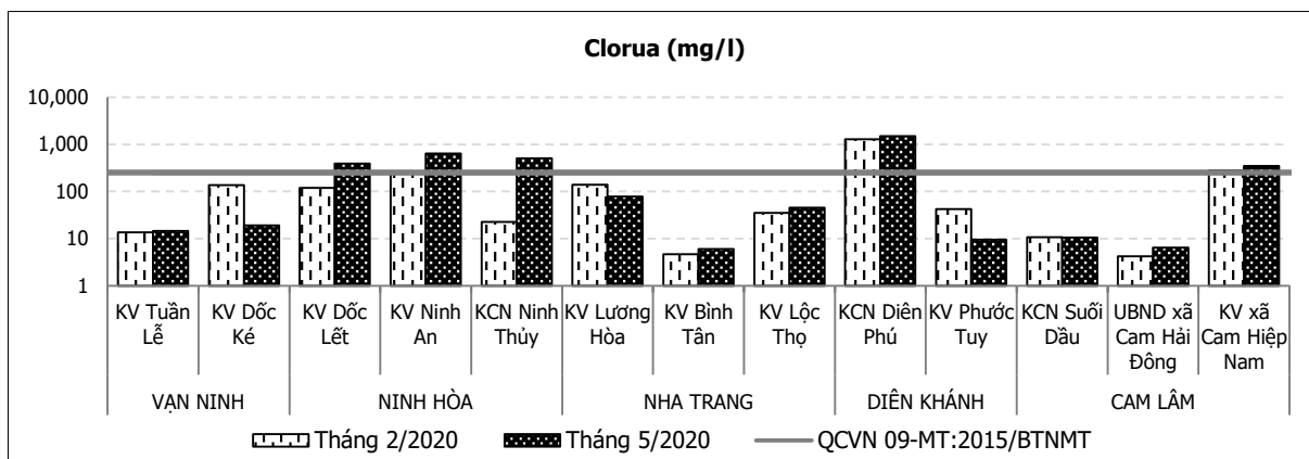
Biểu đồ 2.13. Diễn biến hàm lượng clorua trong nước dưới đất 6 tháng đầu năm 2020
