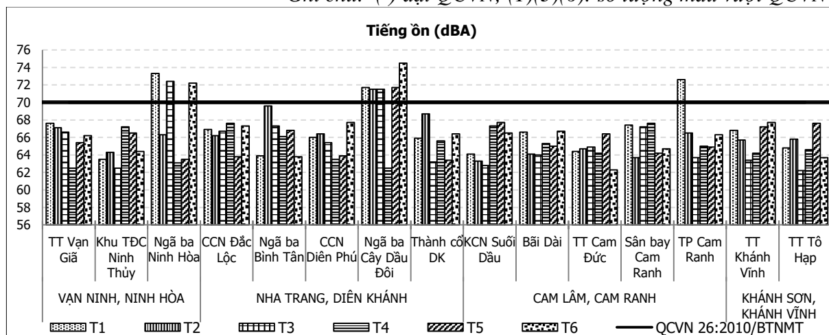
Biểu đồ 2.1. Diễn biến tiếng ồn 6 tháng đầu năm 2020
