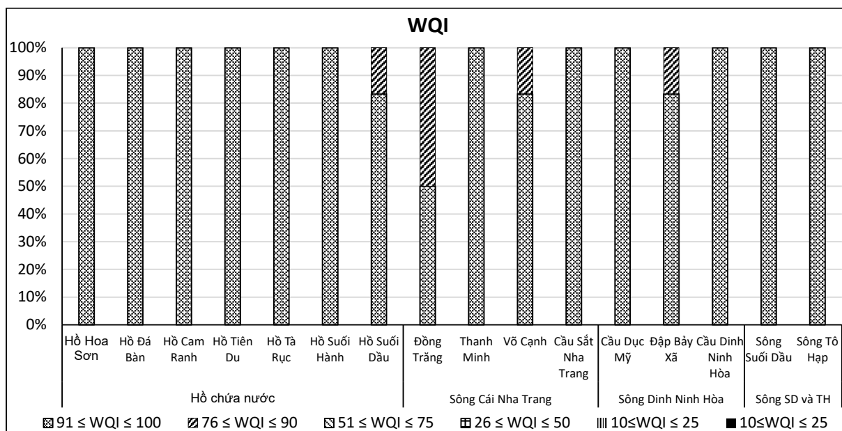
Biểu đồ 2.10. Chất lượng nước mặt theo chỉ số WQI 6 tháng đầu năm 2020
