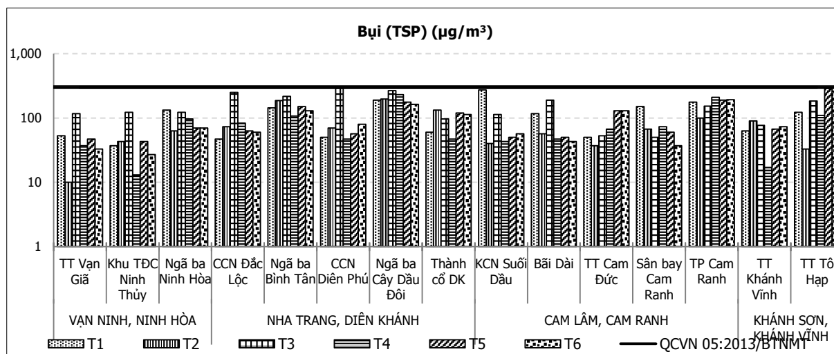
Biểu đồ 2.2. Diễn biến nồng độ bụi (TSP) 6 tháng đầu năm 2020
