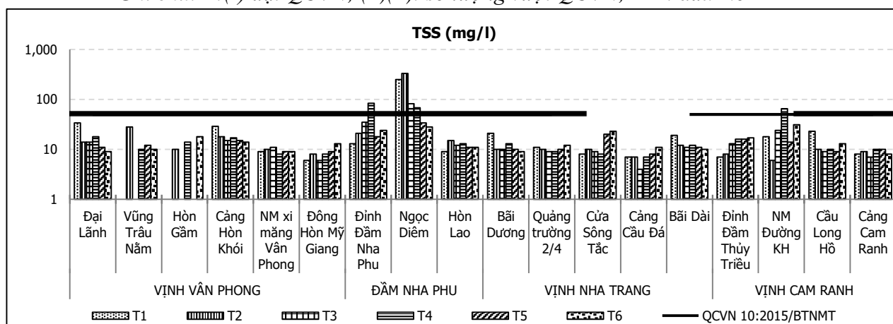
Biểu đồ 2.19. Diễn biến giá trị TSS trong nước biển ven bờ vùng 6 tháng đầu năm 2020
