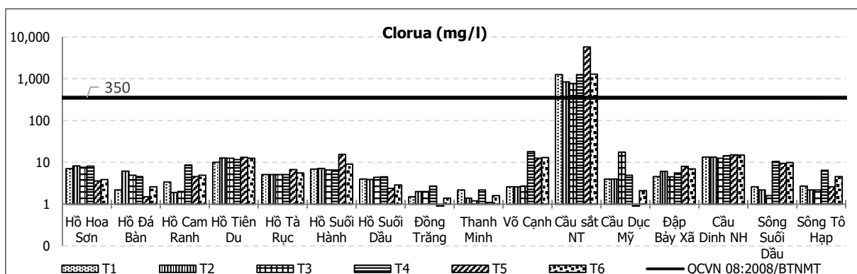
Biểu đồ 2.8. Diễn biến hàm lượng Clorua tại các hồ chứa và sông suối 6 tháng đầu năm 2020
